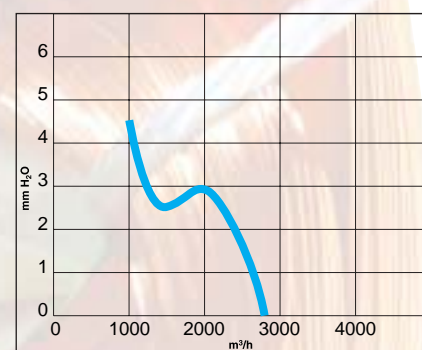
8 poli / poles
