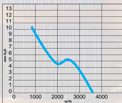
6 poli / poles
